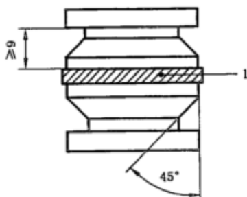
图 2 标准试样
